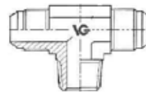
ADAT. A "T" M. JIC- M. NPT AL PIEDE BRANCHTEE JIC - NPT
