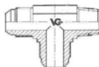
ADAT. A "T" M. JIC- M. BSPT AL BRACCIO RUN TEE JIC - BSPT
