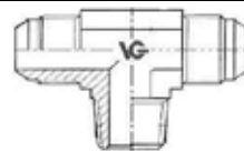
ADAT. A "T" M. JIC- M. BSPT AL PIEDE BRANCH TEE JIC - BSPT
